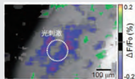
マウス小脳内在ニューロンの光刺激(白円)後に観察された、ニューロン集団(プルキンエ細胞)における応答(青)
