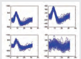
側坐核ニューロンの活動電位波形
