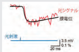
ニューロン(プルキンエ細胞)活動のイメージング(赤)と電気生理学的記録(黒)
